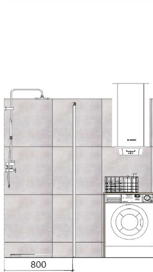
ŚCIANA B
